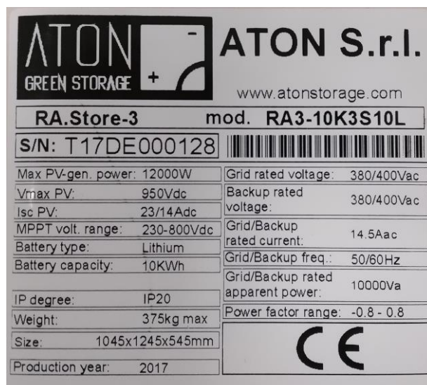
Figura 7 - Targhetta di identificazione
