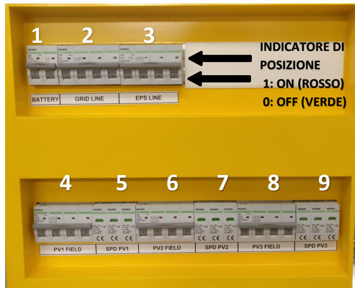
Figura 3 - Frontale quadro elettrico
