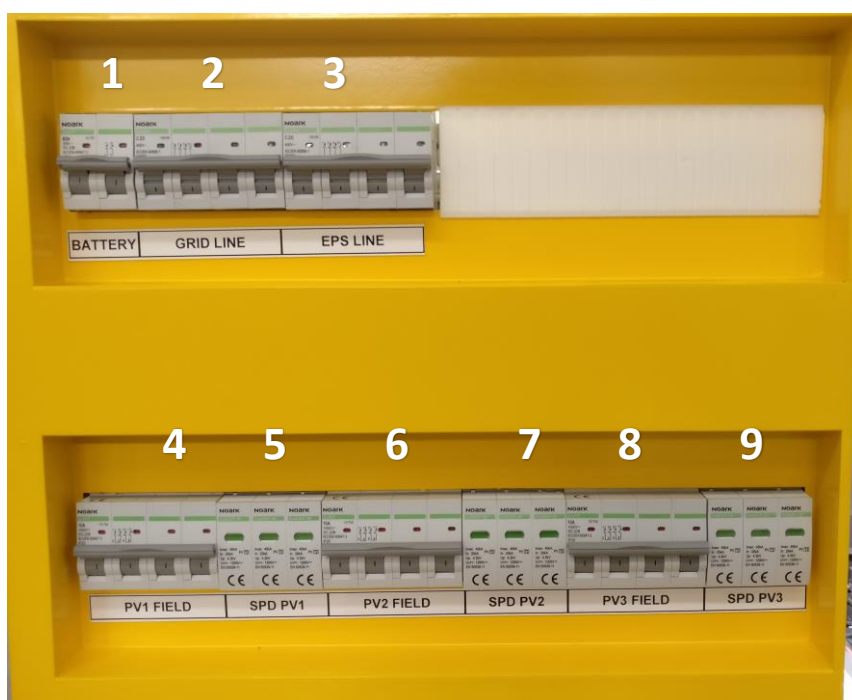
Figura 28 - Frontale quadro elettrico RA.Store-3
